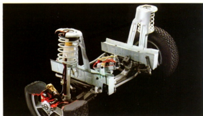
Vorderachse
