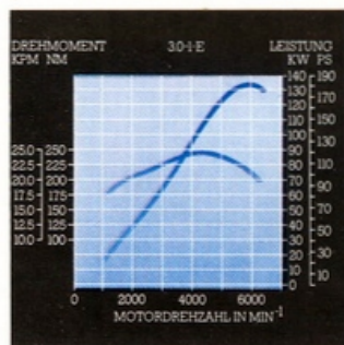
Leistungs-/Drehmoment-Kurve
