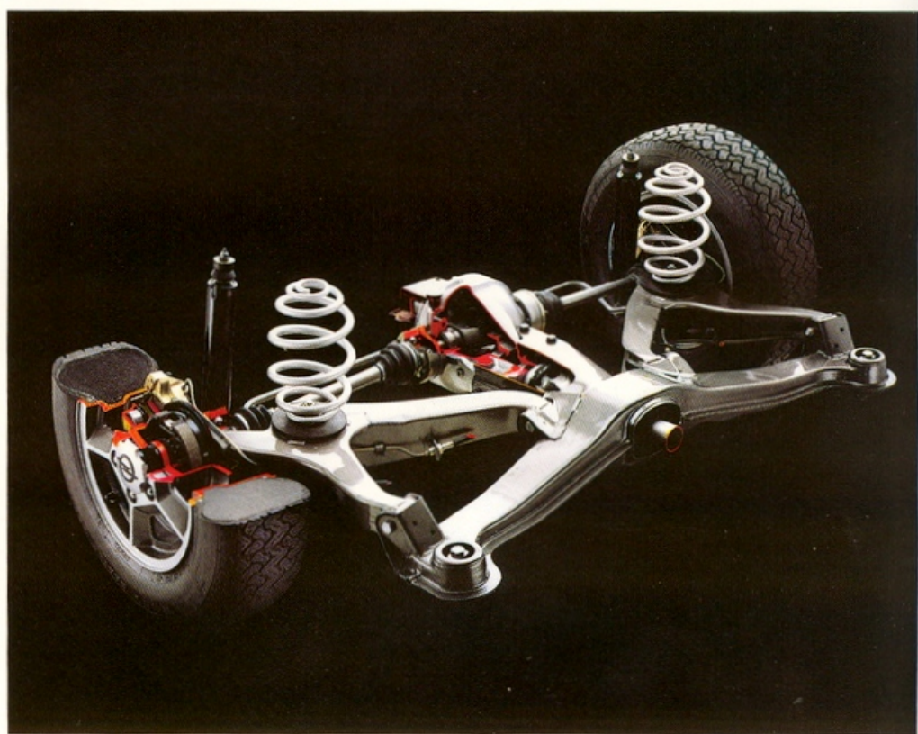
Schräglenker-Hinterachse
